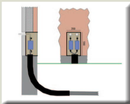
Principskitse for indføringsskab standard-model: H: 590 - B: 350 - D: 200
