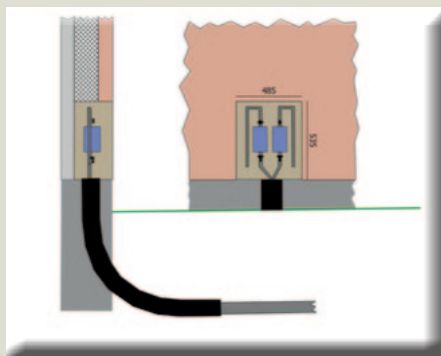
Principskitse for indføringsskab Videbæk-model: H: 535 - B: 485 - D: 200
